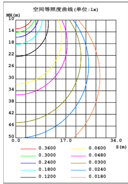
Courbe de Lux distance
